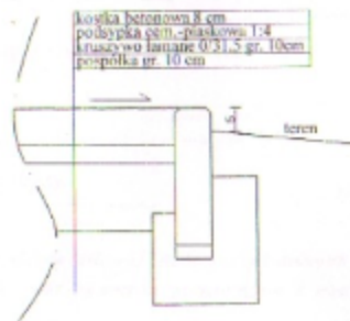
Szczegół chodnika wyniesienie względem terenu +5 cm
